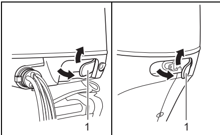
1. Hakenhebel
