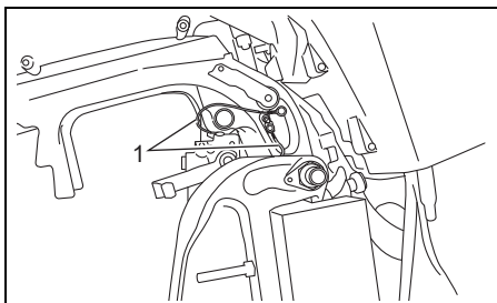
1. Verbindungskabel (DF90AWQH)
