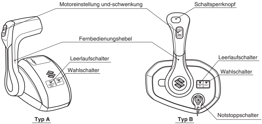
FERNBEDIENUNGSGEHÄUSE (OPTION)
