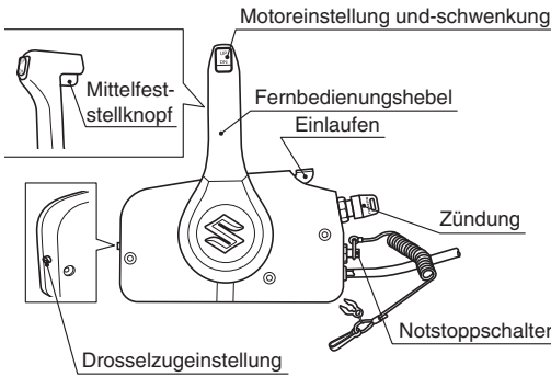
FERNBEDIENUNGSGEHÄUSE ZUR SEITENMONTAGE
