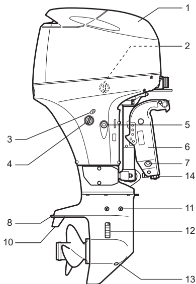
DF40AT/40AST/50AT/60AT
