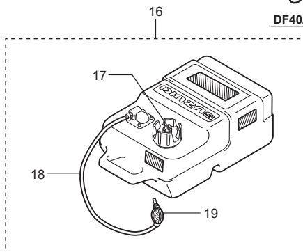
DF40AT/40AST/50AT/60AT
