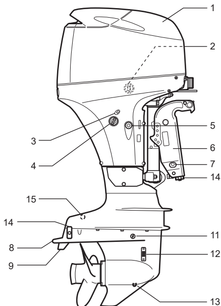
DF40ASVT/60AVT
