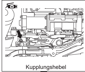
Kupplungshebel
