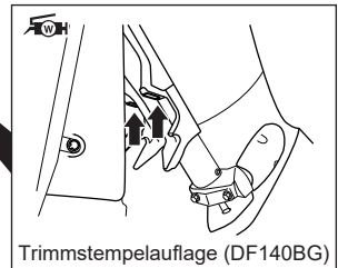
Trimmstempelauflage (DF140BG)
