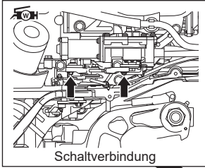
Schaltverbindung
