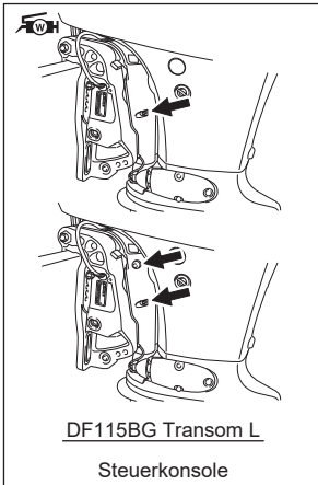
Schaltverbindung
