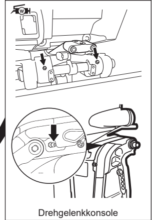
Drehgelenkkonsole
