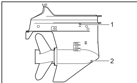
1. Entlüftungsöffnungsschraube/Entlüftungsöffnung 2. Getriebeöl-Ablassschraube/Getriebeöl-Ablassöffnung
