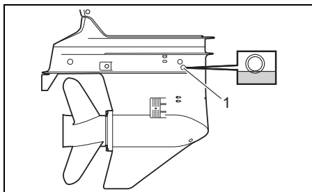
1. Getriebeöl-Kontrollschraube/Getriebeöl-Pegelöffnung
