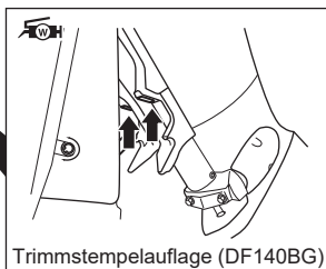
Trimmstempelauflage (DF140BG)
